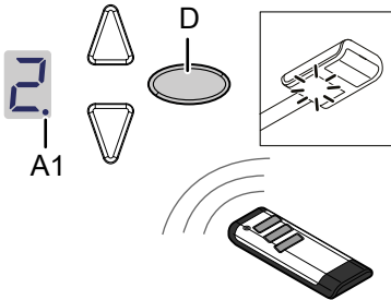
Abb. 10: Lichtfunktion für den Handsender programmieren
