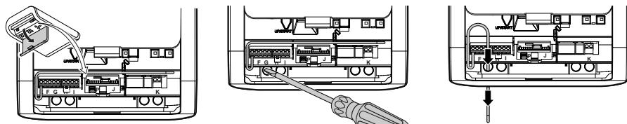
Fig. 8: Tilslutning af antenne
