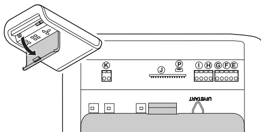
Fig. 7: Ouverture du couvercle de la tête de commande et d'entraînement
