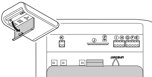
Abb. 7: Abdeckung des Antriebskopfes öffnen
