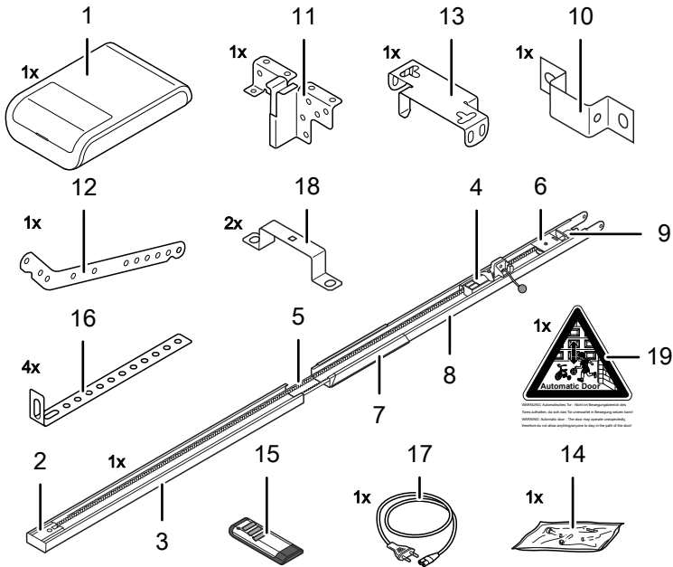
Afb. 4: Leveringsomvang
