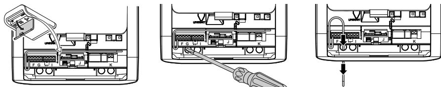
Fig. 8: Poser l'antenne
