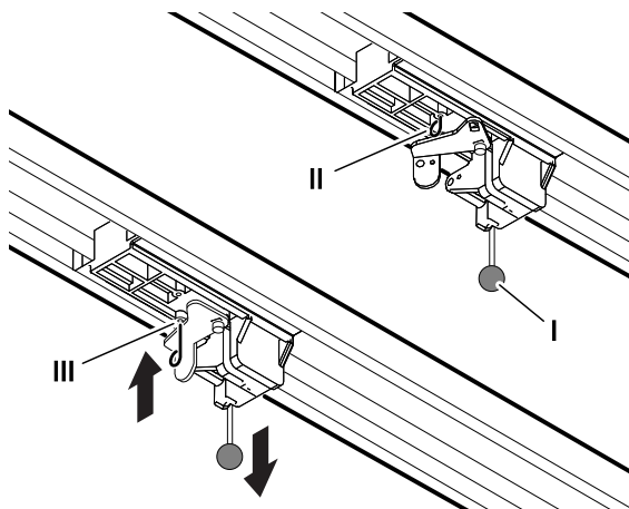
Fig. 16: Déverrouillage et verrouillage de l'entraînement
