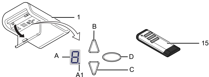
Fig. 2: Betjeningselementer
