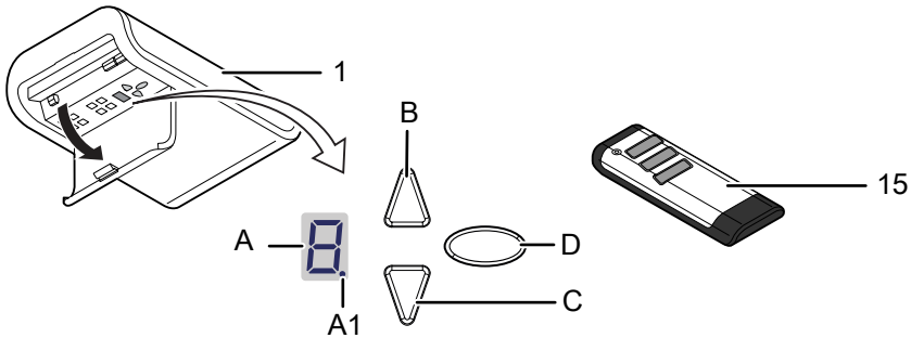
Abb. 2: Bedienelemente
