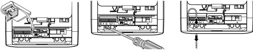
Abb. 8: Antenne verlegen
