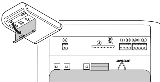
Fig. 7: Åbning af aktuatorhovedets dæksel
